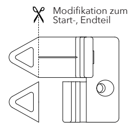
Teilsicht-Verschraubung bei End- und Startdiele
