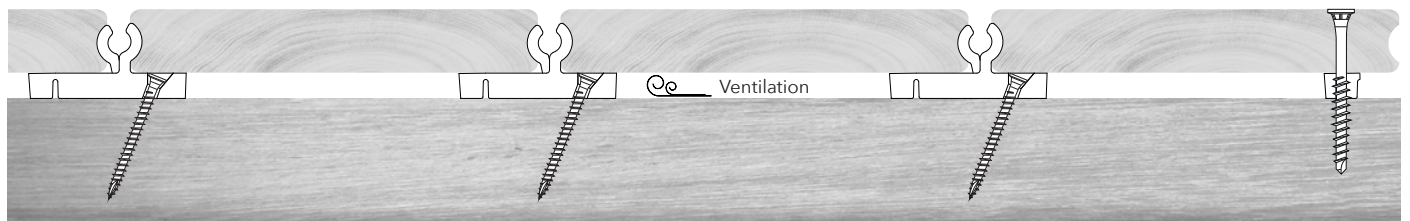
Teilsicht-Verschraubung bei End- und Startdiele
